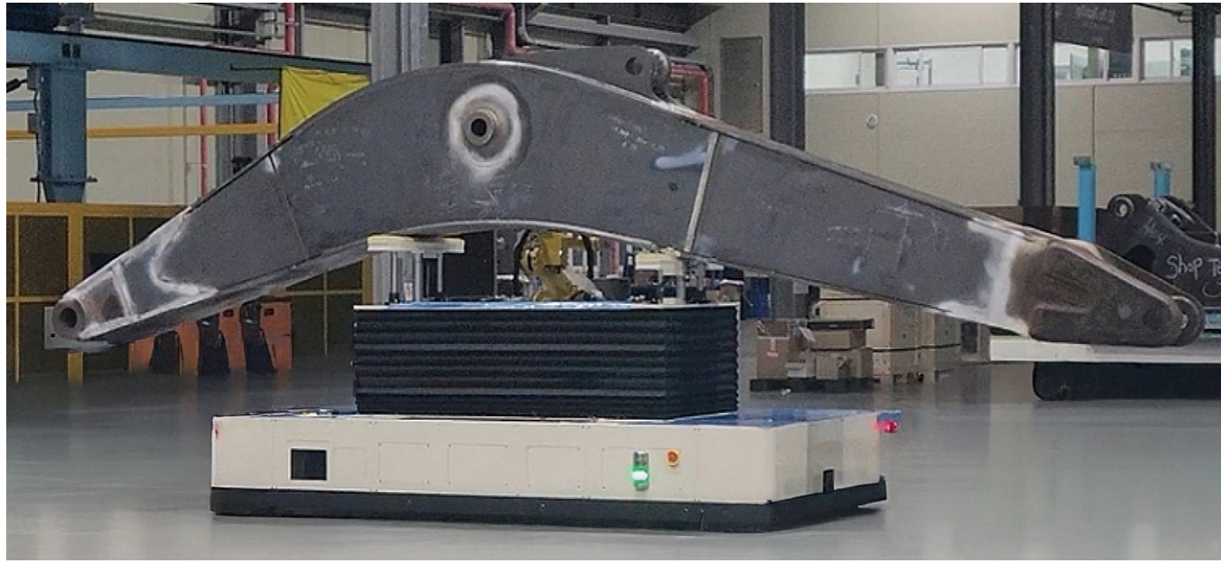
사례 4 H사 5ton 굴착기 붐 이송 AMR
